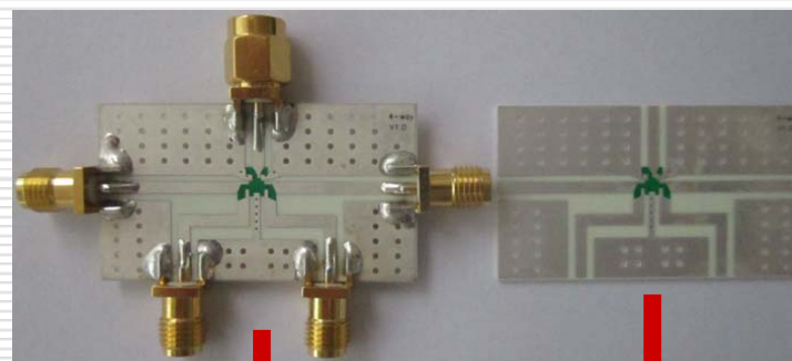
4 way 0°Power Divider
