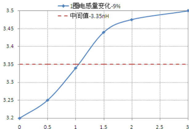
电感量 VS 铝芯旋出高度
