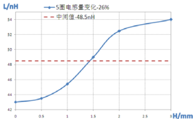
电感量 VS 铝芯旋出高度
