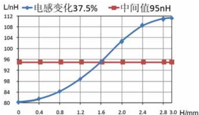
电感量 VS 铝芯旋出高度
