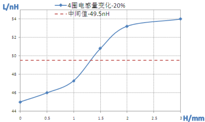
电感量 VS 铝芯旋出高度
