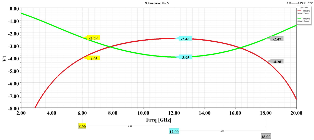
b. 驻波 (6-18GHz)
