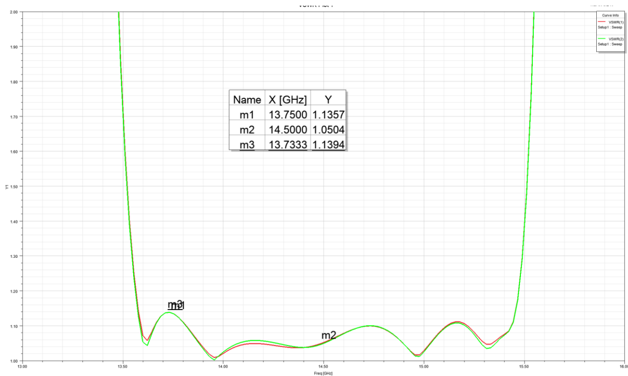
驻波-VSWR
