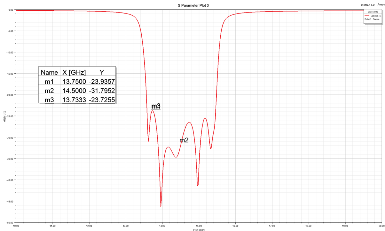
回波损耗-S11
