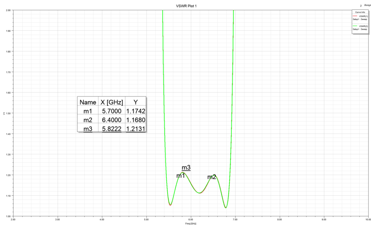
驻波-VSWR
